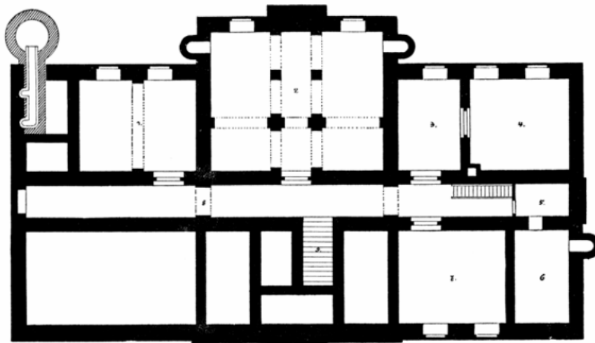
Positiunea interna a localitatilor suterane.
