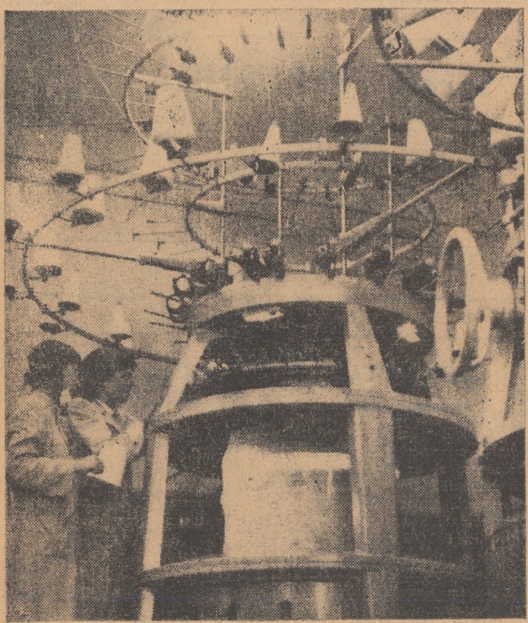
Mașina circulară de tricotat, tip „Harghita”, dispune de 30 sisteme, obținînd în 8 ore o producție de circa 40 kg tricot cu fir de capșeală
