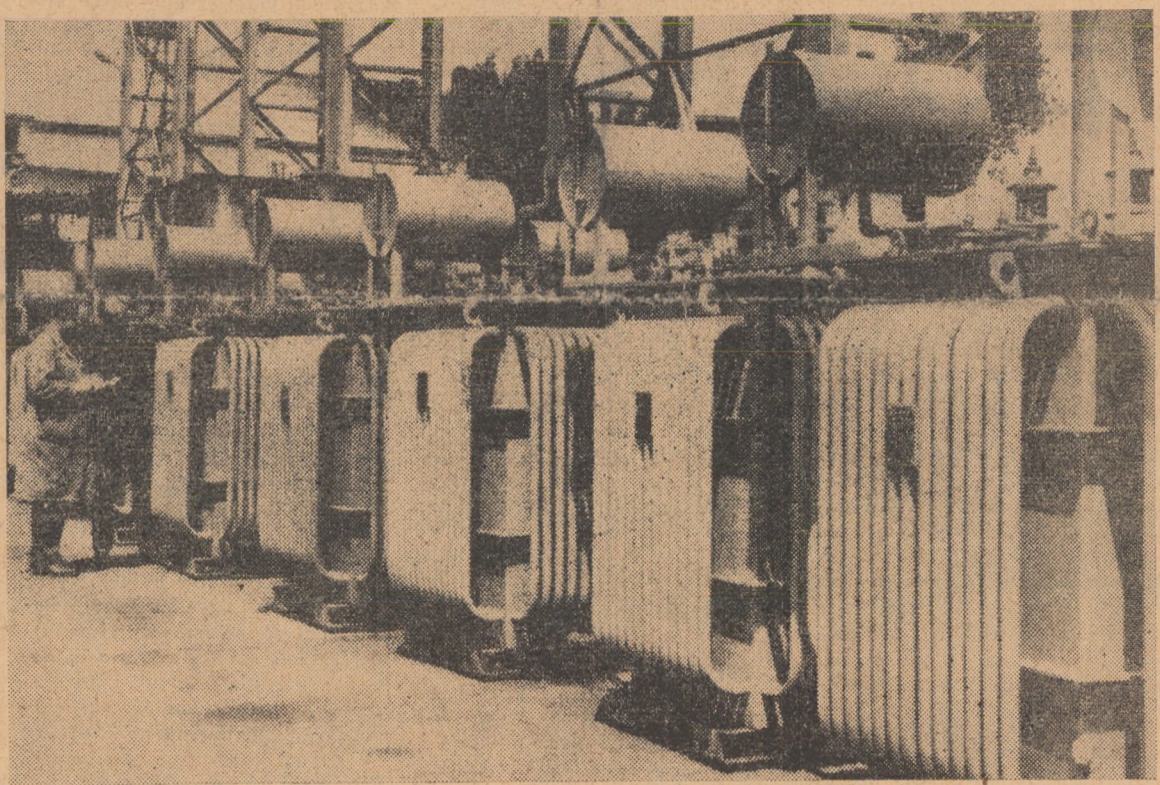
Întreprinderea de electricitate Sibiu, secția de reparat mașini electrice. Un nou lot de bobine de stîngere pentru tratarea neutrului la rețele de 6—15 kV, gata pentru expediere la diferite întreprinderi de electricitate din țară
