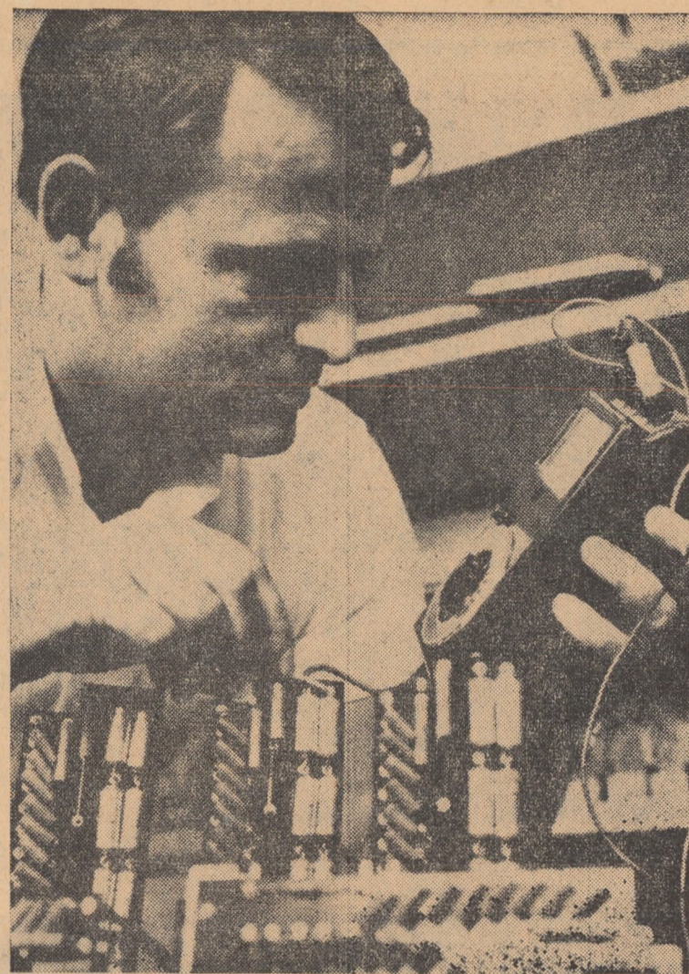
Vasile Bogdan, electrician montator aparate la I.R.M.E. Sibiu verificînd tensiunea de lucru la un megohmmetru tranzistorizat de 2500 V (0—1000 M ), produs al acestei întreprinderi Foto: Fr. NUSS
