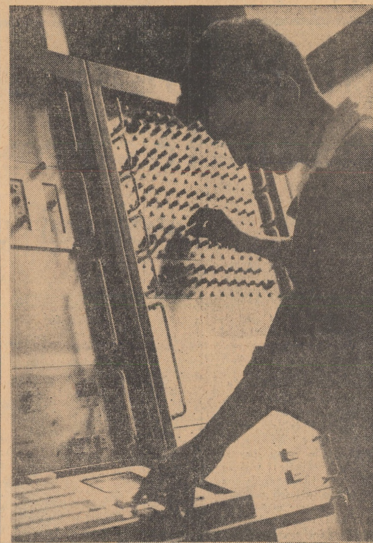
Quantometrul unul din cele mai moderne aparate cu care este dotat laboratorul central al Uzinei chimico-metalurgică din Copsa Mică. Aparatul este folosit la analizele aglomeratului zinc-plumbos și ale zgurei de furnal.
