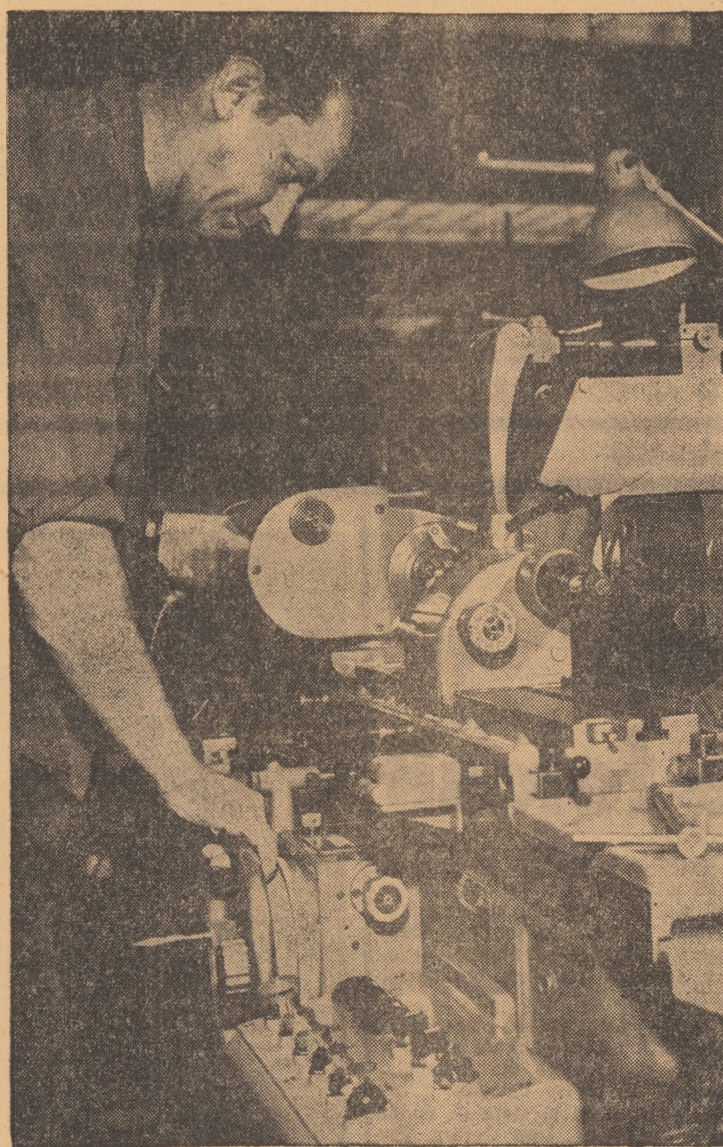
Muncitorul Valerian Perjovski de la „Automecanica” deservind o mașină de verificat profile cu comandă program
