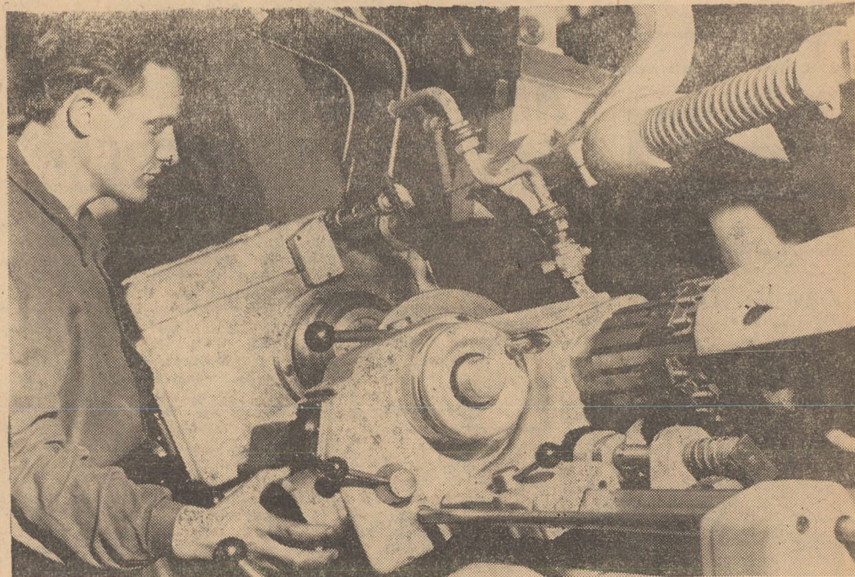
Unul din strungurile revolver cu comandă program de la Uzina mecanică Sibiu. Ținărul Santinel Opris, urmărește cu atenție operațiunile efectuate de noul utilaj
