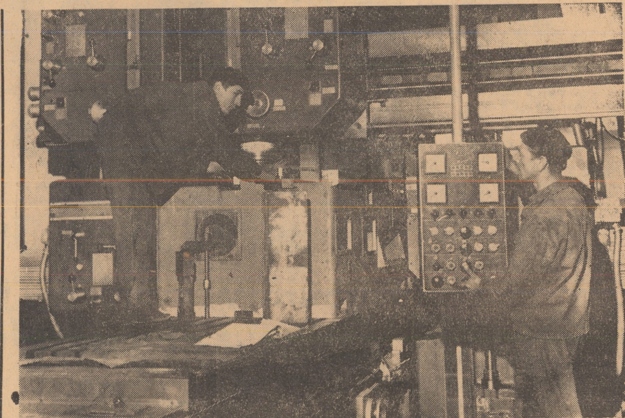
Batiurile și carcassele pentru fereștile automate, produse de Uzina mecanică din Sibiu, sînt prelucrate pe treza portala care efectuează simultan 4 operațiuni de prelucrare. Acest utilaj modern este deservit de Eugen Trigarsky, muncitor cu o înaltă pregătire profesională.
