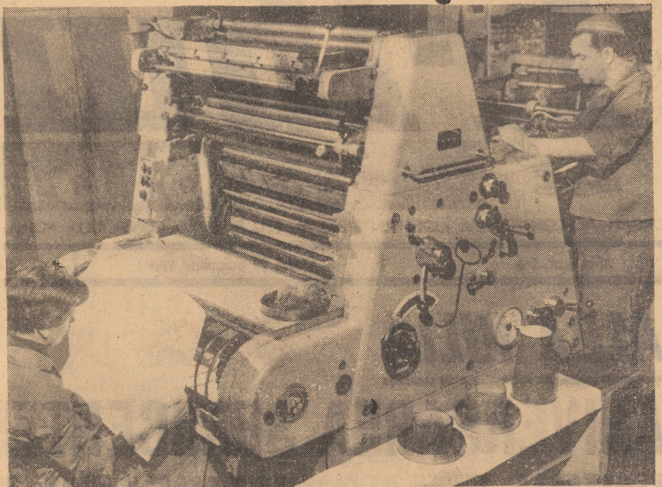
Una din maşinile de tipar plan într-o culoare a secţiei ofset de la Întreprinderea poligrafică Sibiu, la care maşinistul Gîntner Binder şi Hannelore Schneider, muncitoare cu o bună pregătire profesională, execută lucrări de calitate superioară
