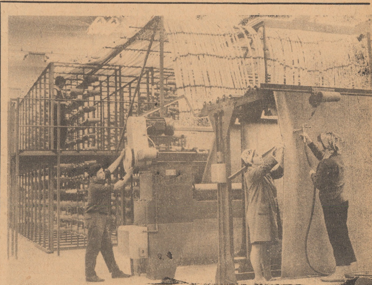
Uzinele Textile Cîsnădie. Mașina „Tufing”, producătoare de covoare, cu o capacitate de 600 m.p. în 8 ore
