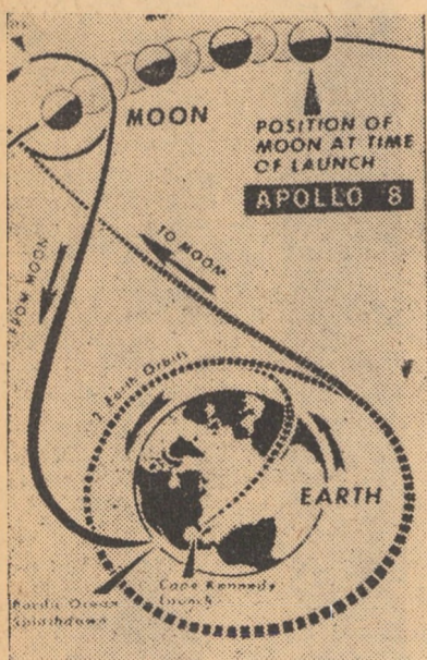
Diagrama apropiatului zbor circumnavigar al navei spațiale americane „Apollo 8”
