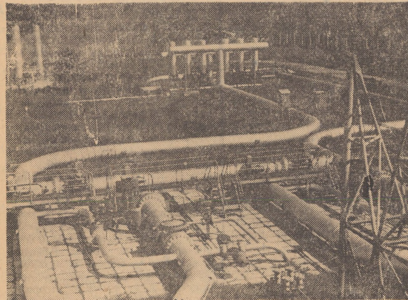
O instalaţie tehnologică exterioră la o staţie de compresoare
