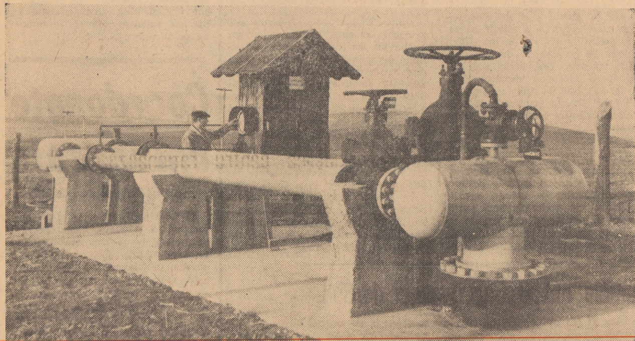
Una din instalaţiile tehnologice folosite în activitatea de transport gaze
