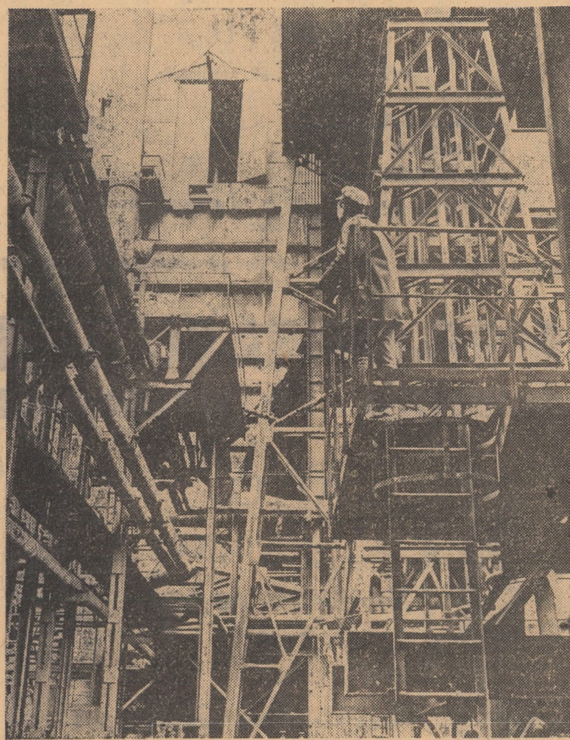
Instalația furnal — anexa șarjare. U.C.M. Copșa Mică.
