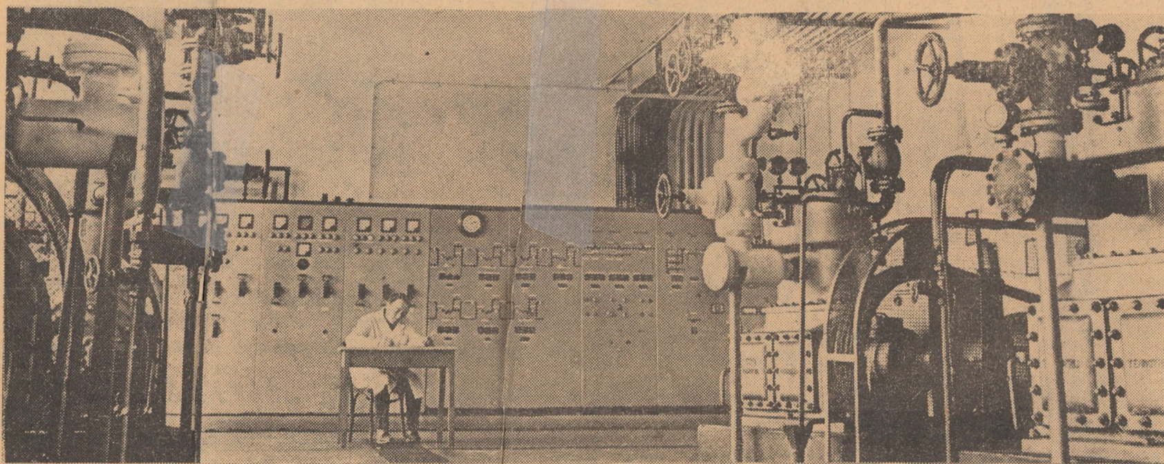
Temperatura scăzută, necesară conservării alimentelor prelucrate de Antrepozitul frigorifer din Sibiu, este obținută de compresoare puternice a căror capacitate însumează 2.300.000 K cal/oră.
