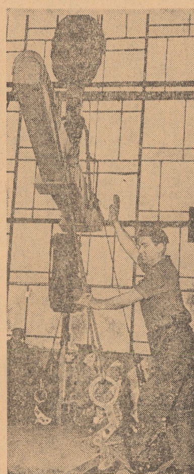
Manevrarea tablei, necesară confecționării viroalelor pentru hidrocentrala Lotru, produse de uzina „Independența” Sibiu, se face cu dispozitive speciale care asigură securitatea muncii.
