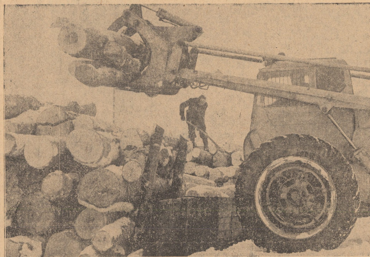
I.F. Sibiu. Sector de industrializare lemnului Tâlmăciu. La rampa de descărcare C.F.R. (I.F.R.O.N.) Incărcător frontal, produs de I.R.U.M. Sibiu
