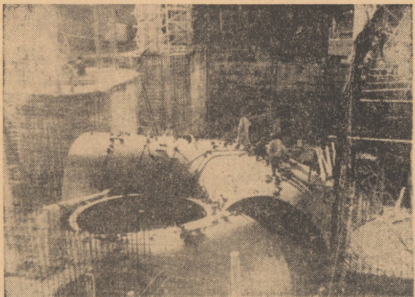
U.R.S.S. În defileul Gevark din R.S.S. Gruzină se află în construcție complexul hidroenergetic de pe riul Ingursk 5 din hidrocentralele acestui complex vor avea o putere de 1 640 000 kW. În fotografie: Aspect de pe șantierul uneia din hidrocentralele complexului
