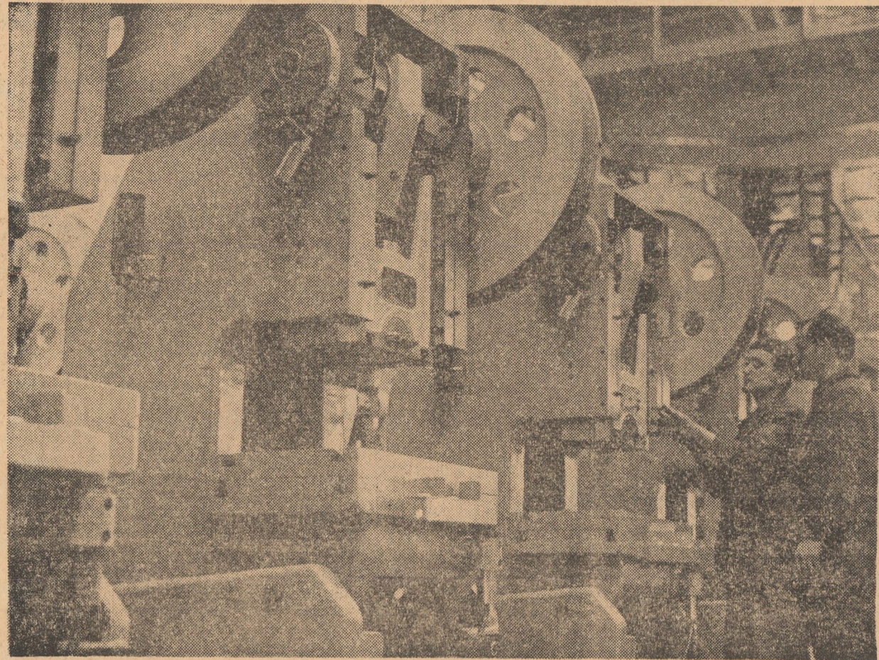
Un lot de prese cu excentric de 40 tone/forță produse de Uzina mecanică Sibiu, care vor fi livrate beneficiarilor de peste hotare
