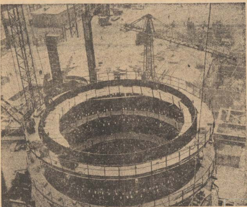
U.R.S.S. În apropierea celui de-al doilea furnal al Uzinei metalurgice din regiunea Kemerovsk se află în construcție un al treilea cuplor cu o capacitate de 3.000 mc, care va fi cel mai mare din țară. Producția anuală a noului cuplor va fi de aproape 2 milioane tone fontă. În foto: pe șantierul celui de-al treilea cuplor
