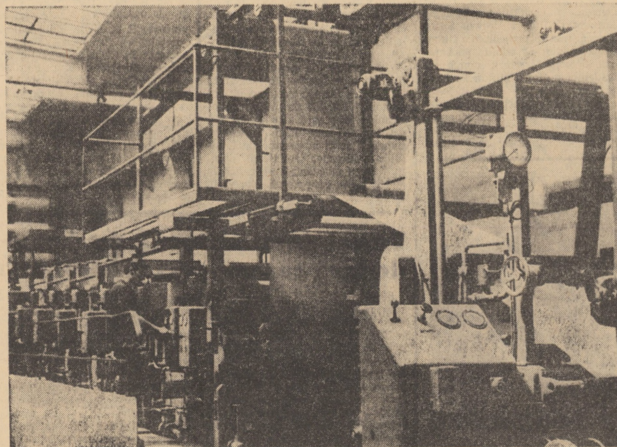
Fixarea coloranților la țesăturile produse de uzina „Tirnavă” Mediaș se face cu ajutorul unei mașini de vaporizare cu o capacitate de 8000 metri liniari în 8 ore
