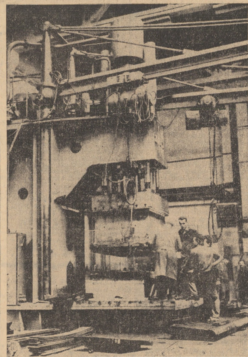
La uzina „Automecanica” Medias o presă hidraulică de 600 tone produce capacele de mare gabarit la cisternele pentru transportul lapteului
