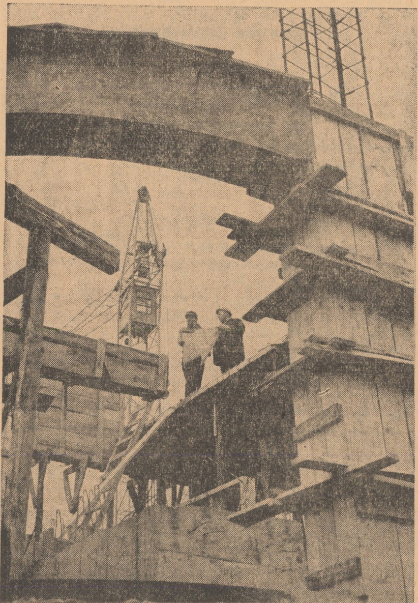
Pe șantierul Casei de cultură a sindicatelor din Sibiu, lucrările s-au început în luna februarie a.c. În prezent construcția este ridicată în roșu (cca. 65 la sută). Se lucrează la turnul scenei și la cel al II-lea etaj pentru acoperirea sălii de spectacole
