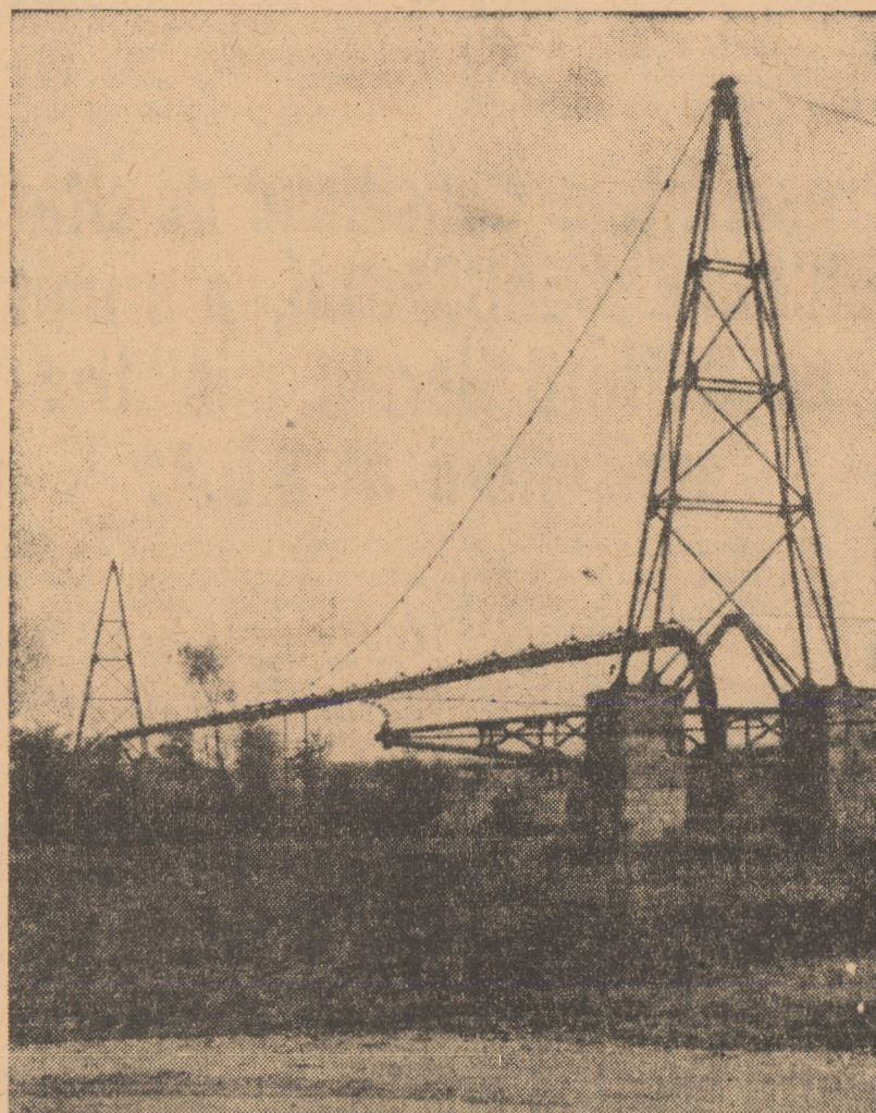
Tip de traversare aeriană suspendată a unei conducte magistrale de transport gaz peste un curs de apă
