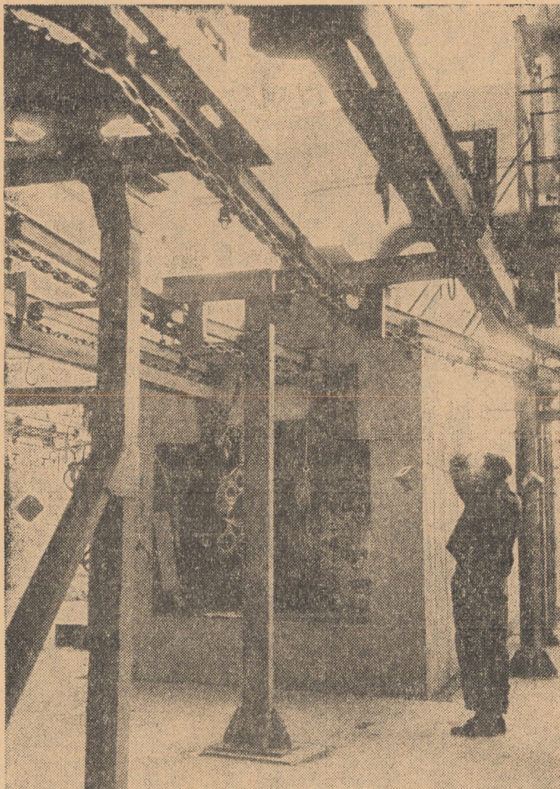
Unul din cele două cupatoare ale noului vopșitor al uzinei „Balanta” Sibiu, dotat cu cite două benzii transportoare care, la fiecare 20 secunde, scot cite o piesă, sau un grup de piese, din cupor
