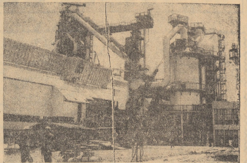
R.S.F. IUGOSLAVIA. În prezent, în apropiere de Belgrad, se află în construcție oțelăria „SMEDEREVO” (din care o mare parte sînt date în funcțiune) care atunci cînd vor fi complet terminate vor produce 2 milioane tone de fier brut anual. În foto: vederea parțială a oțelăriei „SMEDEREVO” de lângă Belgrad
