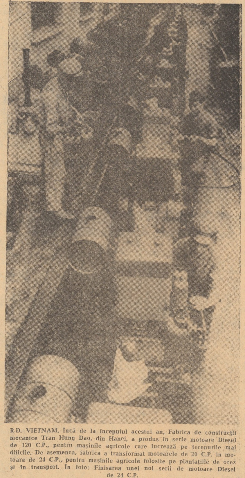
R.D. Vietnam. Încă de la începutul acestui an, fabrica de construcții mecanice Tran Hung Dao, din Hanoi, a produs în serie motoare Diesel de 120 C.P., pentru mașinile agricole care lucrează pe terenurile mai dificile. De asemenea, fabrica a transformat motoarele de 20 C.P. în motoare de 24 C.P., pentru mașinile agricole folosite pe plantațiile de orez și în transport. În foto: Finisarea unei noi serii de motoare Diesel de 24 C.P.
