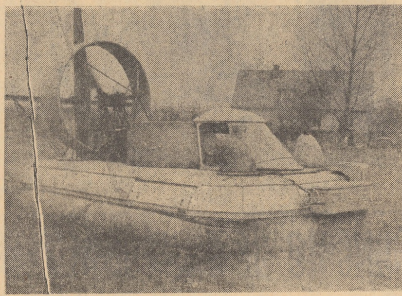
R.P. POŁONA. O echipă de cercetători de la Institutul de mecanizare a agriculturii și de la Institutul de aviație au realizat un prototip al unui vehicul cu pernă de aer „M-6 Ursynow”, primul de acest fel din Polonia și al treilea din lume. Vehiculul va avea o largă întrebuintare în agricultură, va fi folosit în mare măsură la împrăștierea substanțelor protectoare pentru plante și a îngrășămintelor, înlocuind avioanele și vor fi folosite pe terenurile unde celelalte mașini agricole nu se pot deplasa cu ușurință. În foto: noul vehicul cu pernă de aer „M-6 Ursynow” realizat în Polonia
