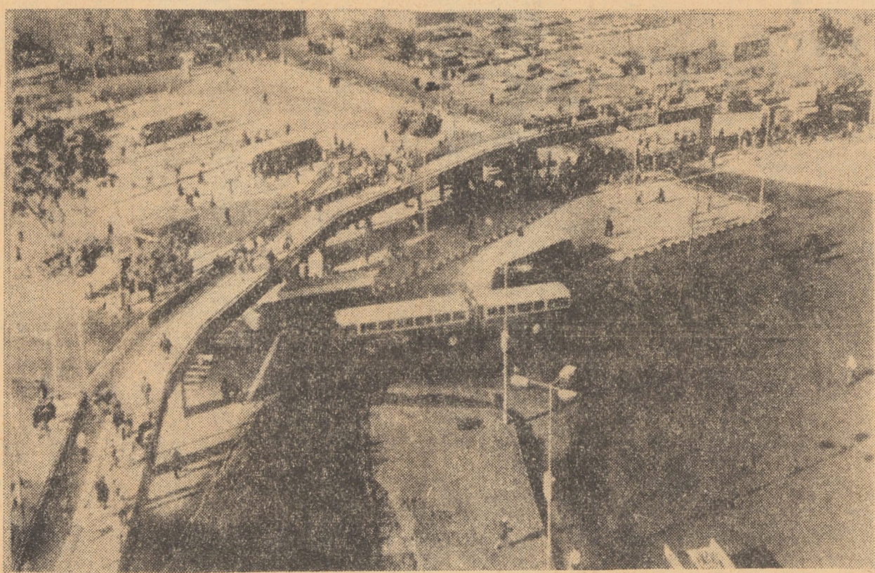
Piața Tahrir din Cairo a ridicat dificile probleme de trafic din cauza numărului mare de perso- ne care o traversau. Soluția a- doptată a fost aceea a construirii unei pasarele pentru pietoni. În foto: Noua pasarelă pentru pietoni din Piața Tahrir din Cairo
