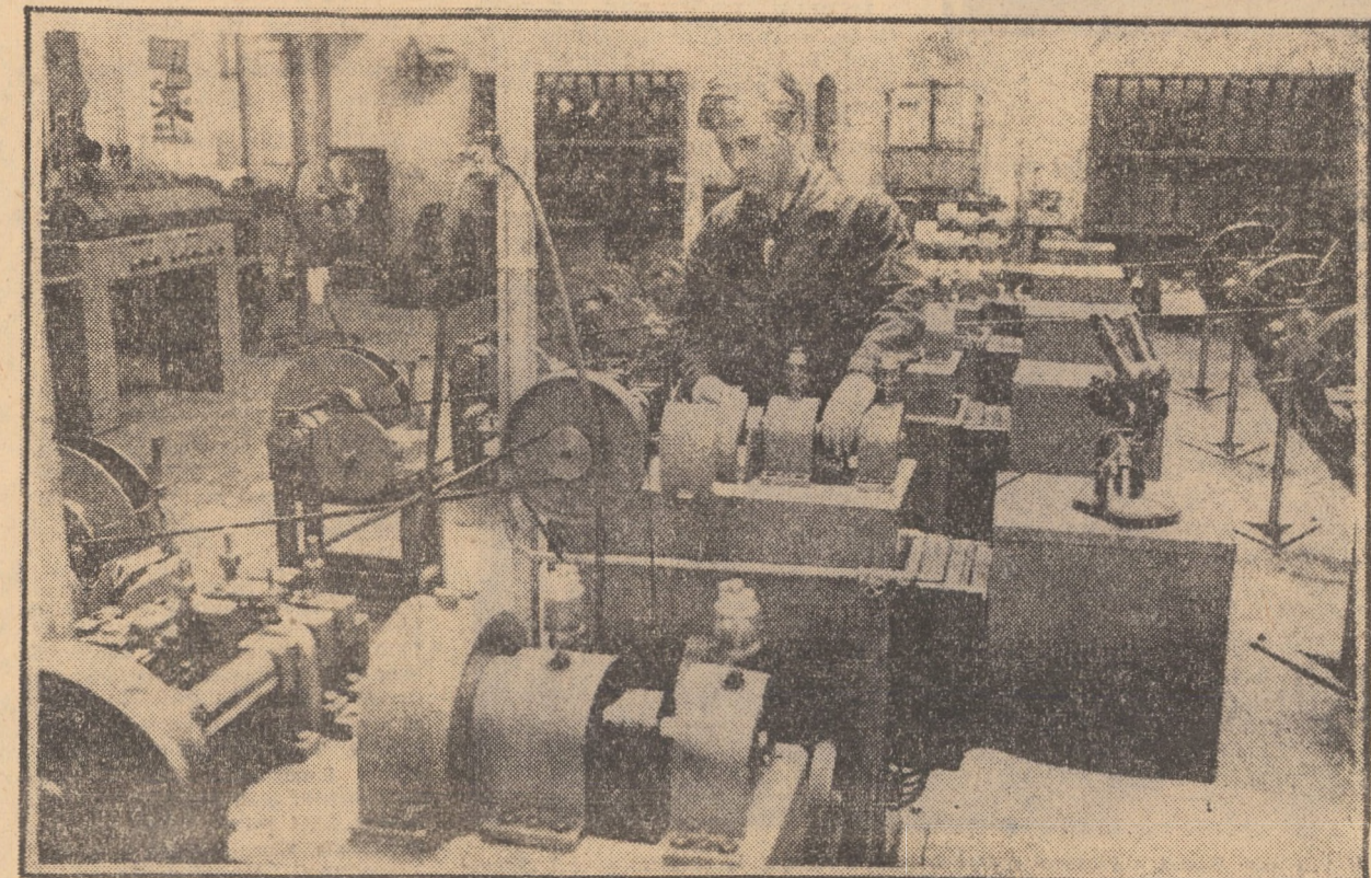
Linia de stîlțat a garniturilor rigide din secția metal de la „Flora” Sibiu, deservită de comunistul Gheorghe Mureșan lăcătus reșor cu o bună pregătire profesională
