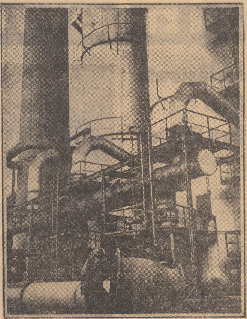
Instalații moderne de preîncălzirea aerului la furnale la U.M.M.N. Copșa Mică Foto: HORST BUCHFELNER
