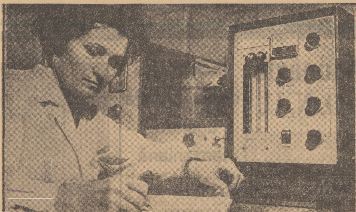
Spectrometru cu absorbție atomică — aparat de înaltă precizie și rapiditate cu care este înzestrat laboratorul central de la U.M.M.N. Copsa Mică, este utilizat pentru determinarea tuturor metalelor fără să fie necesară o prealabilă separare. În fotografie: laboranta Georgeta Gîrlea deservind acest aparat. Foto: FRED NUSS
