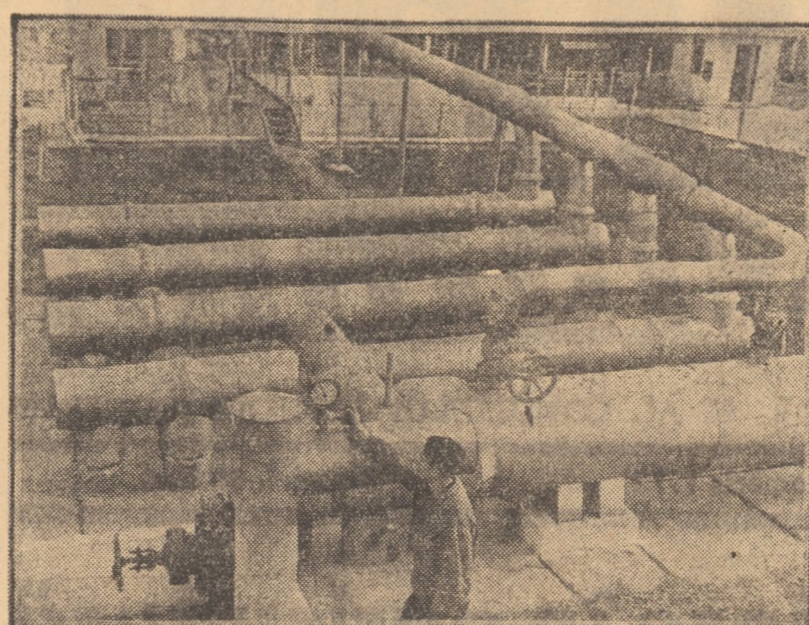
Instalație de încălzire și uscare a gazului metan a întreprinderii conducte magistrale din cadrul Centralei Industriale gaz metan Medias
