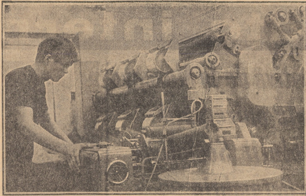
Filatura de lână sempleplănată a Uzinei Textile Cîsnădie. Cardă cu cap laminar — utilaj de mare productivitate, deservit de acenul anului I. Florin Nicolaescu
