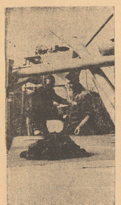
R.P. POLONĂ. La Institutul de cercetări chimice al tehnologiei cărbunului și petrolului lampant din Wrocław s-a găsit o nouă metodă de brichetare a cărbunului și de echipare a stațiilor de brichetare. În foto: Prototipul echipamentului de brichetare construit la mina „Sosnowiec” unde s-au și efectuat teste semitehnice.
