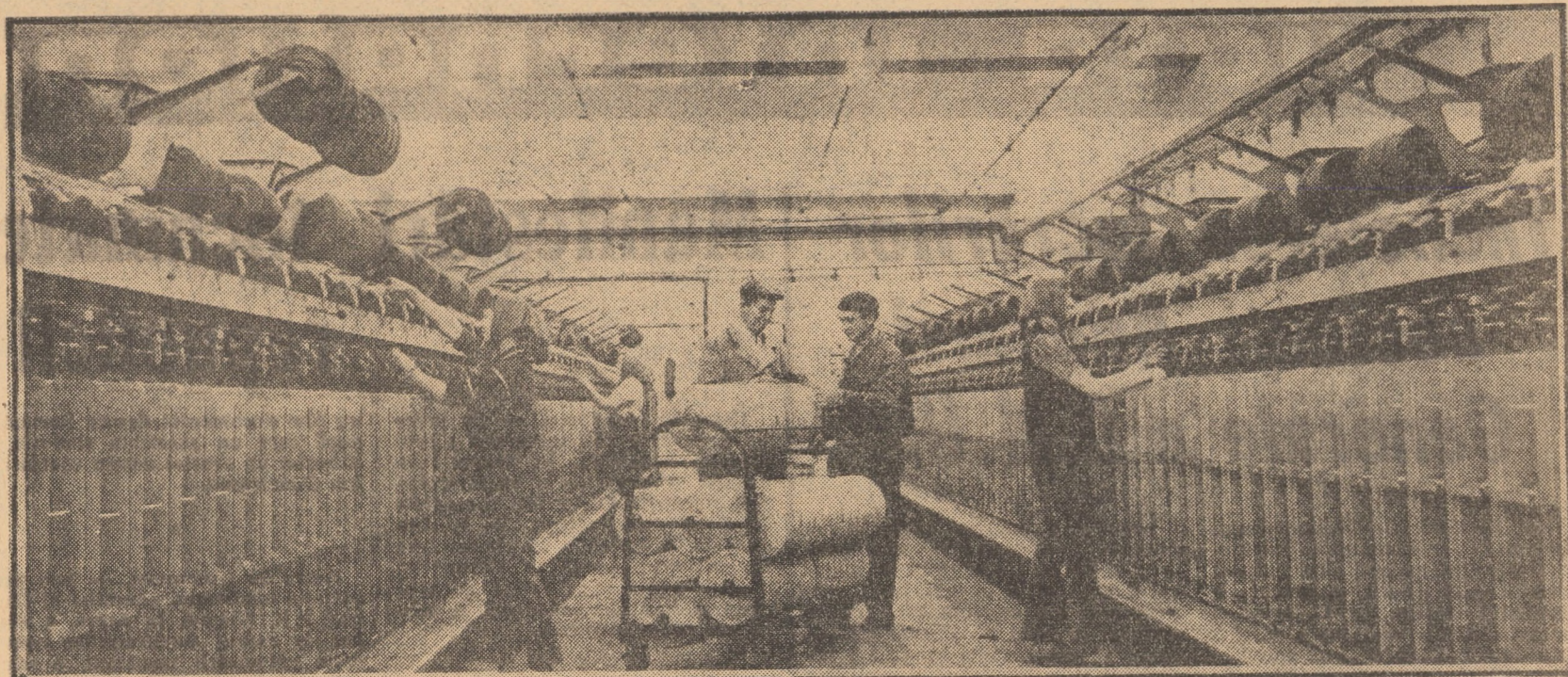
De curînd, în secția filatură a fabricii „Progresul” din Orlat, au fost puse în funcțiune două mașini cu inele cu 168 fusuri fiecare, utilaje moderne, de mare productivitate. În foto: Gheorghe Ilina, șef secție și Ioan Grăf, ajutor maestru (mijloc), analizînd calitatea firelor
