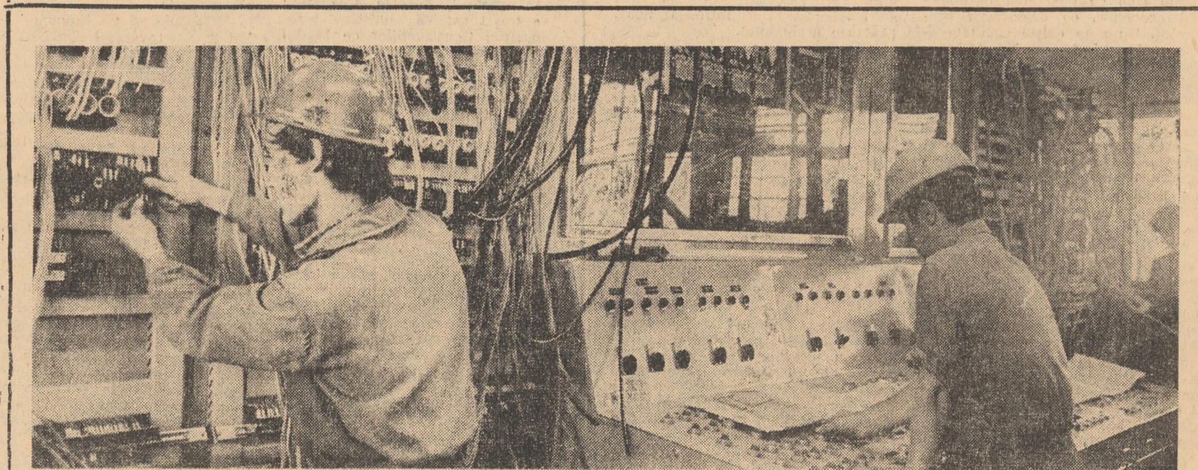
La „Independența” II din Sibiu se lucrează intens la montarea instalațiilor complexe în cabina de comandă a stației automate de preparat amestec de formare pentru fontă. Foto: HORST BUCHHEINER
