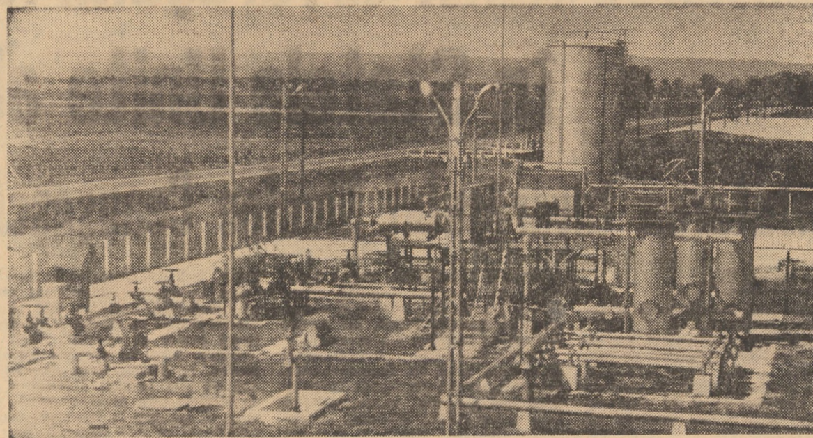
Stația de tratare gaze Homocia - vedere spre panoul de măsură și instalația de uscare
