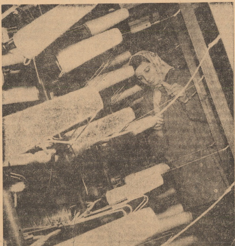
Din sutele de bobine ale ramei de alimentare, (în foto) firul „se scurg” spre mașina „Tufing” — utilaj modern de mare capacitate, producător de covoare la întreprinderea „Dumbrava” din Sibiu
