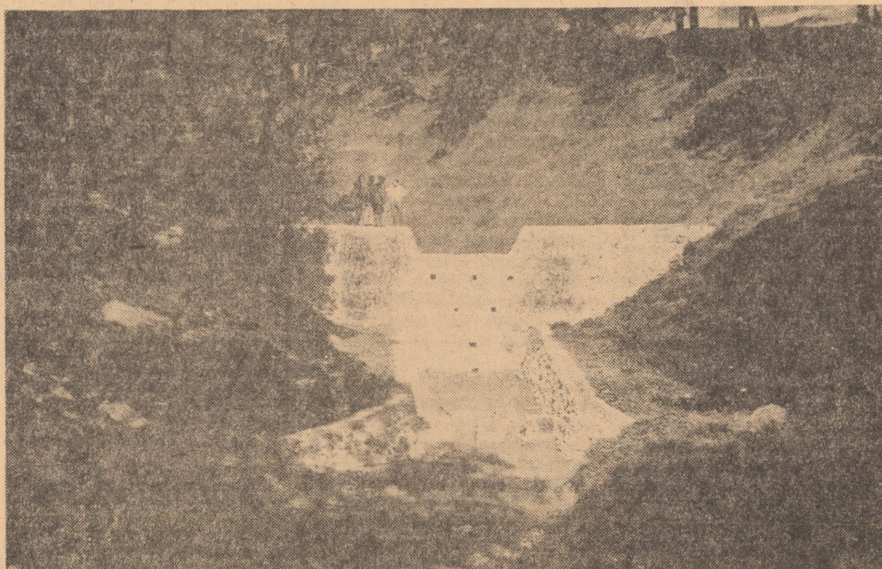
Oficiul de îmbunătățiri funciare din cadrul Direcției generale județene a agriculturii, execută ample lucrări de combatere a eroziunii. În fotografie: Baraj de zidărie, în bazinul hidrografic Dumbrăveni
