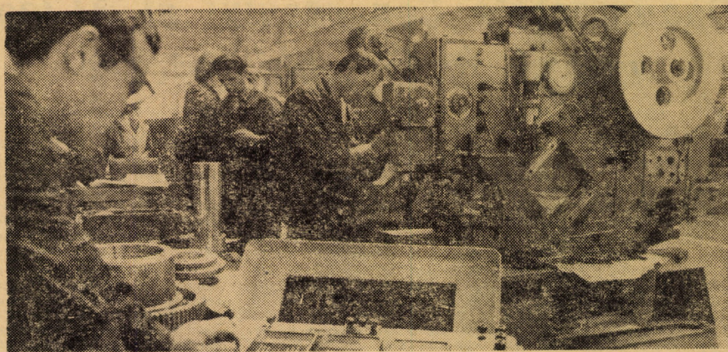
Verificarea parametrilor funcționali la presele cu excentric în hala de montaj a întreprinderii mecanice Sibiu. Foto: FRED NUSS
