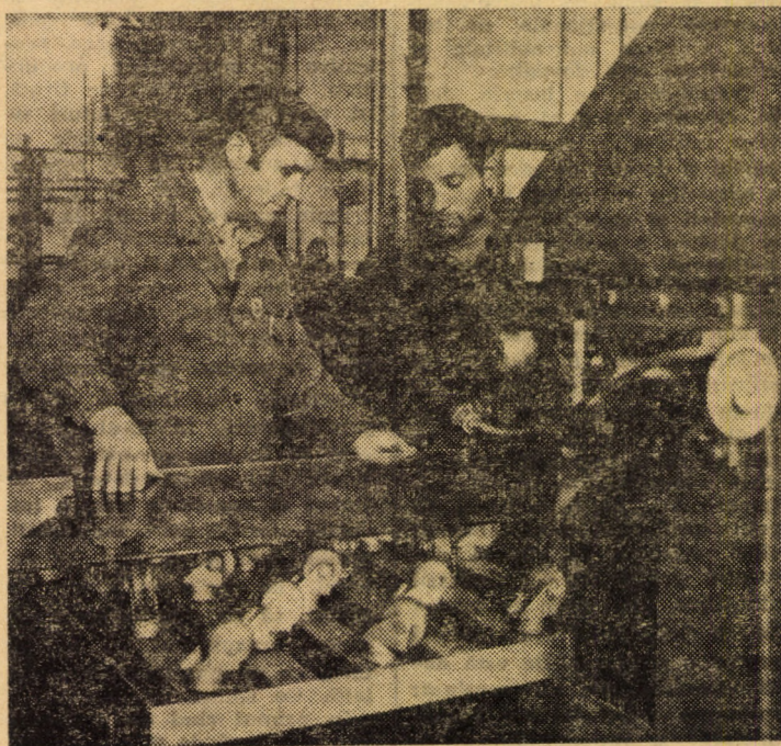
Autoutilarea — preocupare de prim ordin la Fabrica de geamuri Mediaș, în foto: mașină de șlefuit geam, realizată în atelierele proprii.
