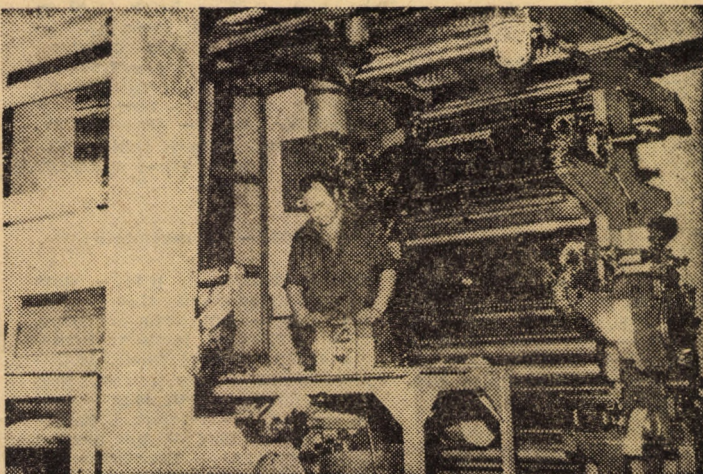
Mașina de imprimat din secția termoplast de la IMIX Agnita.
