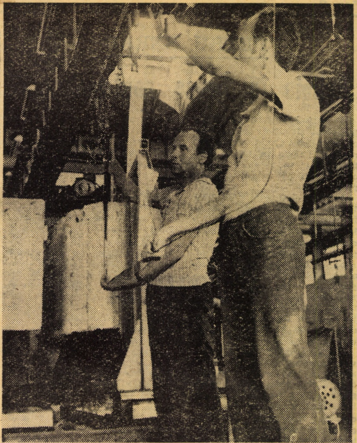
Fabrica de geamuri Mediaș. Linia de securizare a parbrizelor pentru autocamioanele Roman-Diesel Foto: HORST BUCHFELNER
