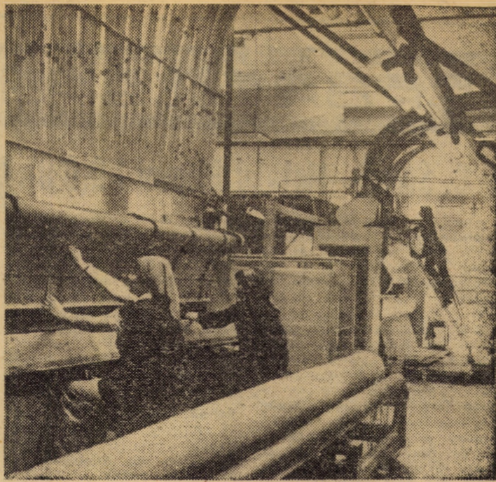
Întreprinderea „Dumbrava” Sibiu. Mașina de țesut covor plușat, tip „TUFFED”. La acest utilaj modern operația de țesut și formarea plușului este concomitentă. Foto: FRED NUSS
