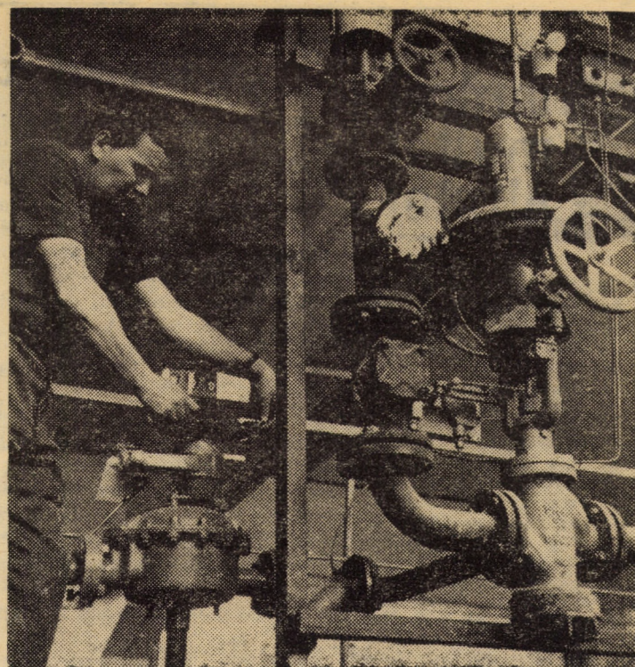
Instalații moderne de dozare în noua tăbăcărie minerală a Întreprinderii „13 Decembrie” Sibiu
