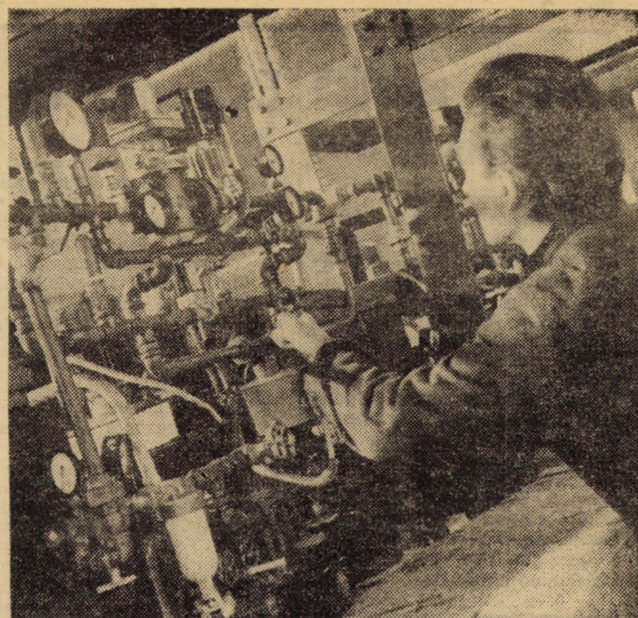
Noutăți la „Flamura roșie” Sibiu? Da, între multe altele, instalația de distribuție a liniei automate de cromare „GALVAPOL”, recent dată în funcțiune
