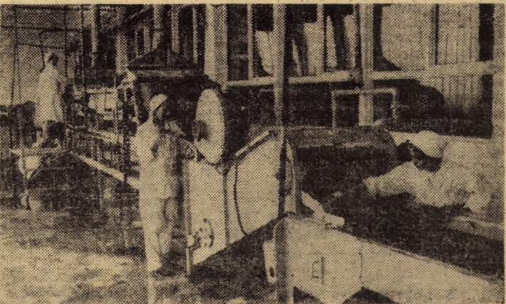
Linia de conservat fasole prin frig cu o capacitate de 500 kg/oră — utilaj modern în cadrul sectorului semipreparate al Fabricii „Frigoriferul” din Sibiu Foto: FRED NUSS
