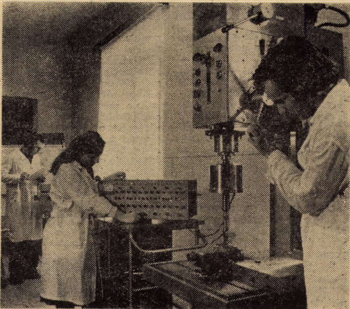
La Facultatea de mecanică Sibiu a fost adaptat un dispozitiv de măsurare a forței axiale și de torsiune
