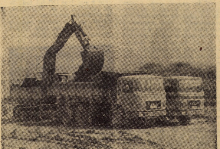
Autobasculante grele din Sibiu la punctul de încărcare de pe șantier Foto: I. SORESCU
