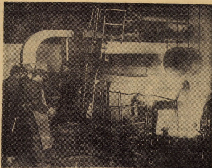
Elaborarea unei șarje de oțel la turnătoria întreprinderii „Independența” Sibiu Foto: FR. NUSS
