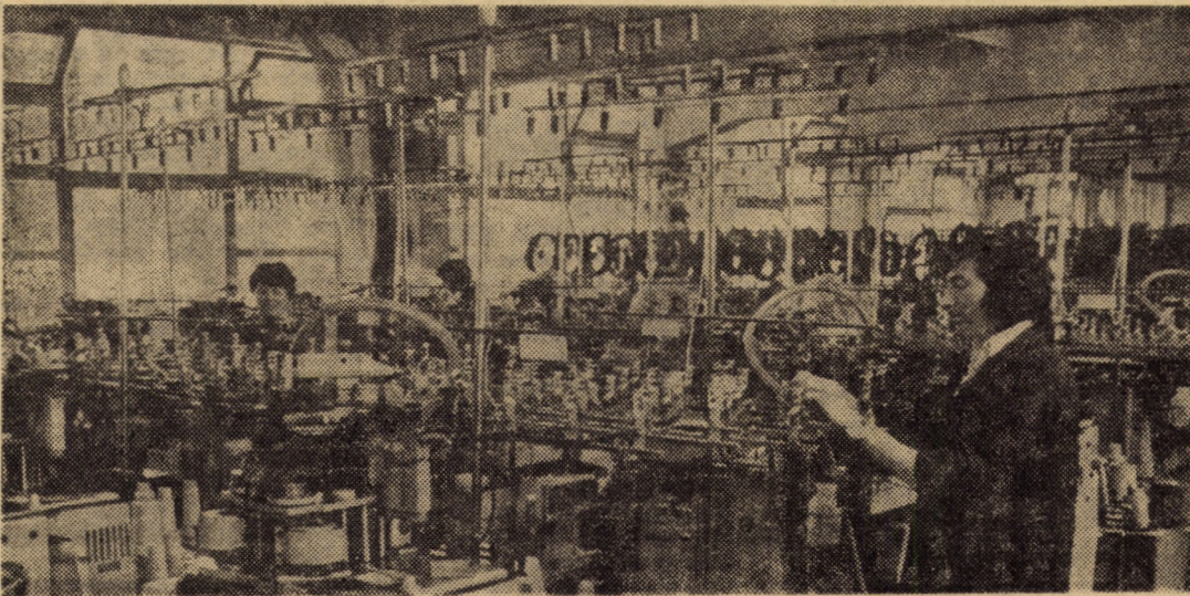
În sala mașinilor de tricatat a Întreprinderii de mînuși și ciorapi Agnita
