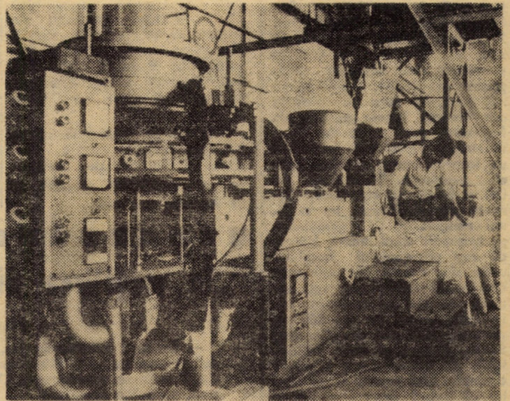
Mașină de extrudat folii din polietilenă — utilaj de mare productivitate, complet automatizat, din atelierul prelucrări mase plastice de la IMIX Agnita
